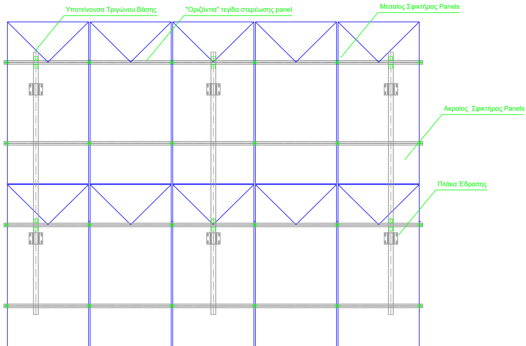
ΚΑΤΟΨΗ ΒΑΣΗΣ - ΔΙΑΤΑΞΗ 2x5 Portrait
